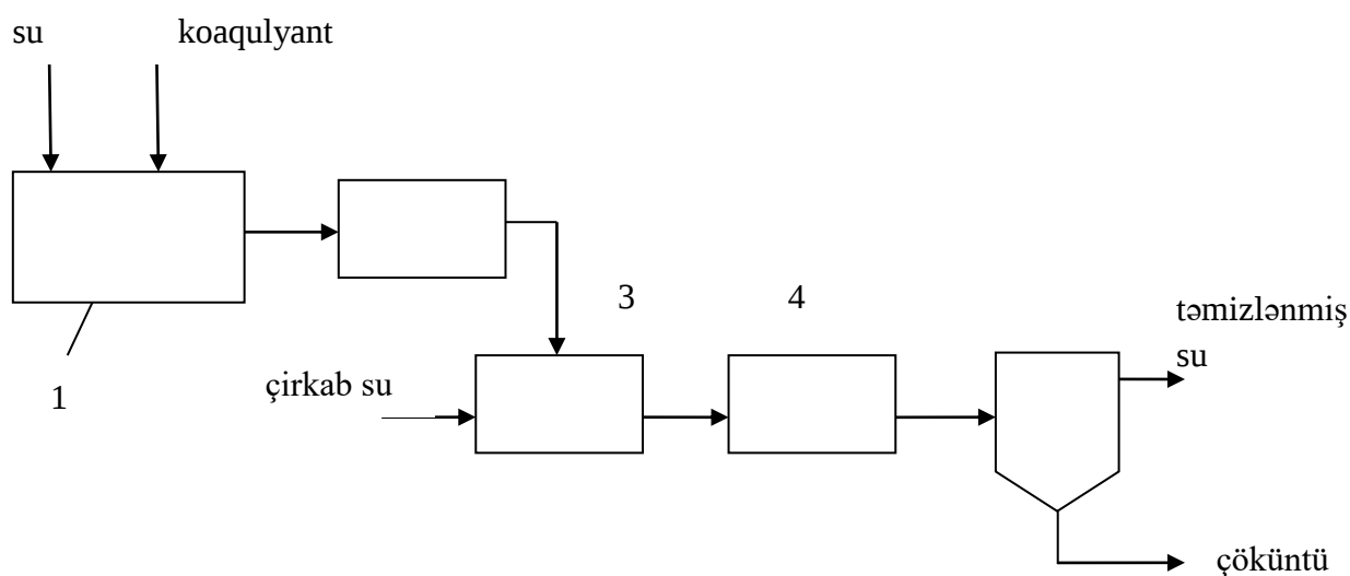
Sxem 2.4 Çirkab suların koagulyasiya üsulu ilə təmizlənməsi
