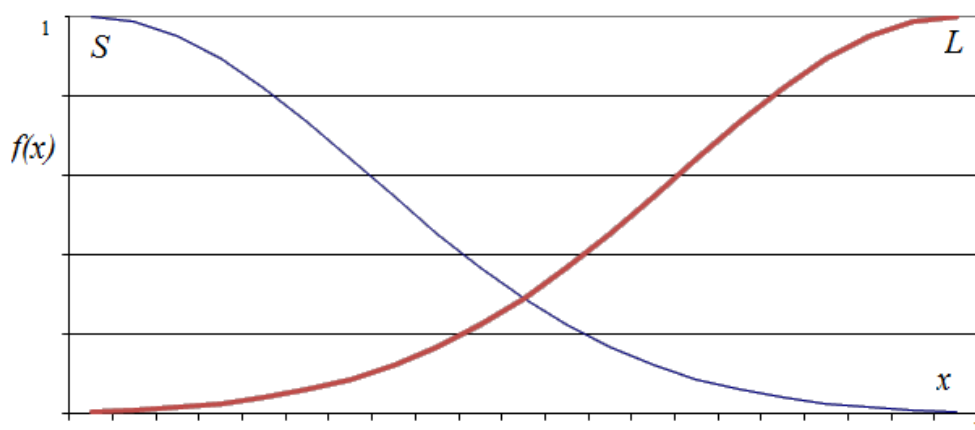
Рис. 3.4: Функции принадлежности комплементарной нечёткой связи
