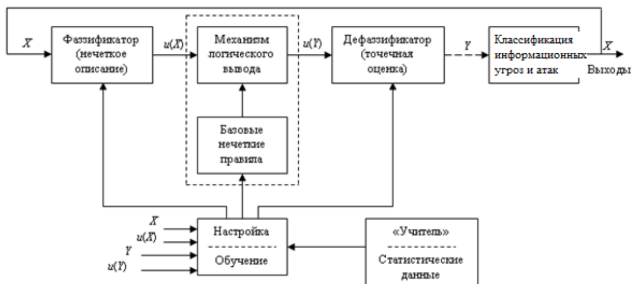
Рис. 2.3: Классификация информационных угроз на основе адаптивной системы нечёткого вывода
