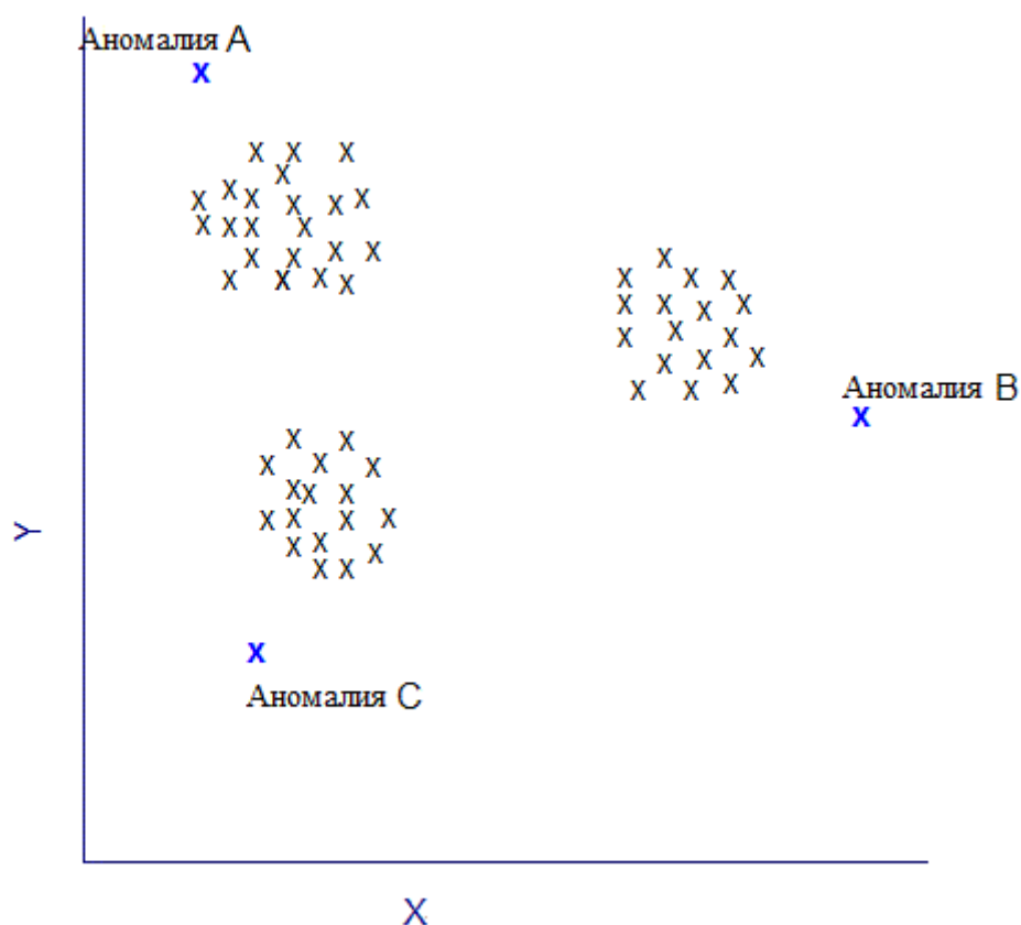
Рис. 7. Аномалии
