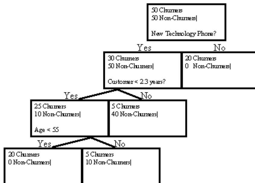
Рис.5. Дерево Решений
