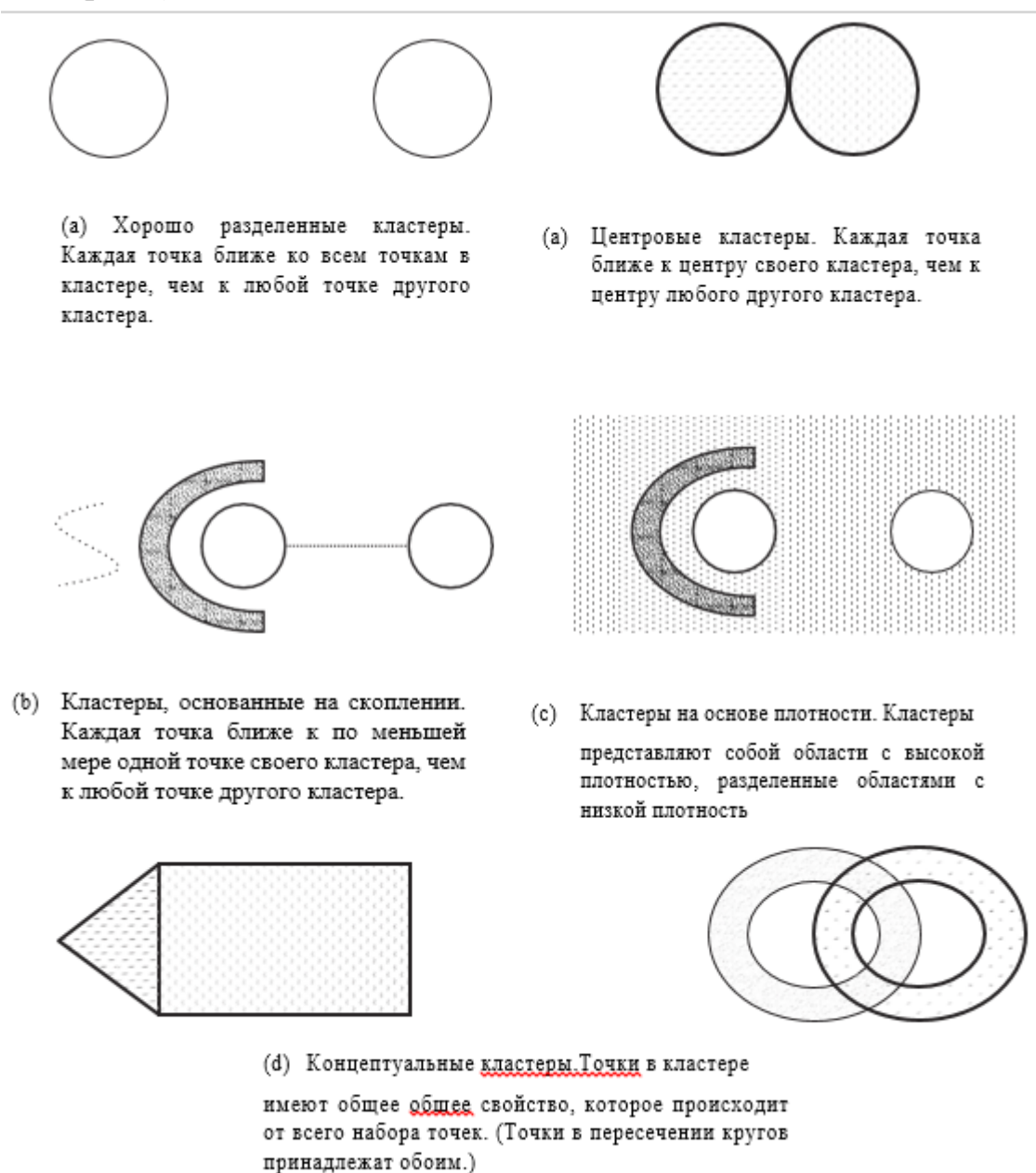
Рис.8. Различные типы кластеров, показанные множествами двумерных точек
