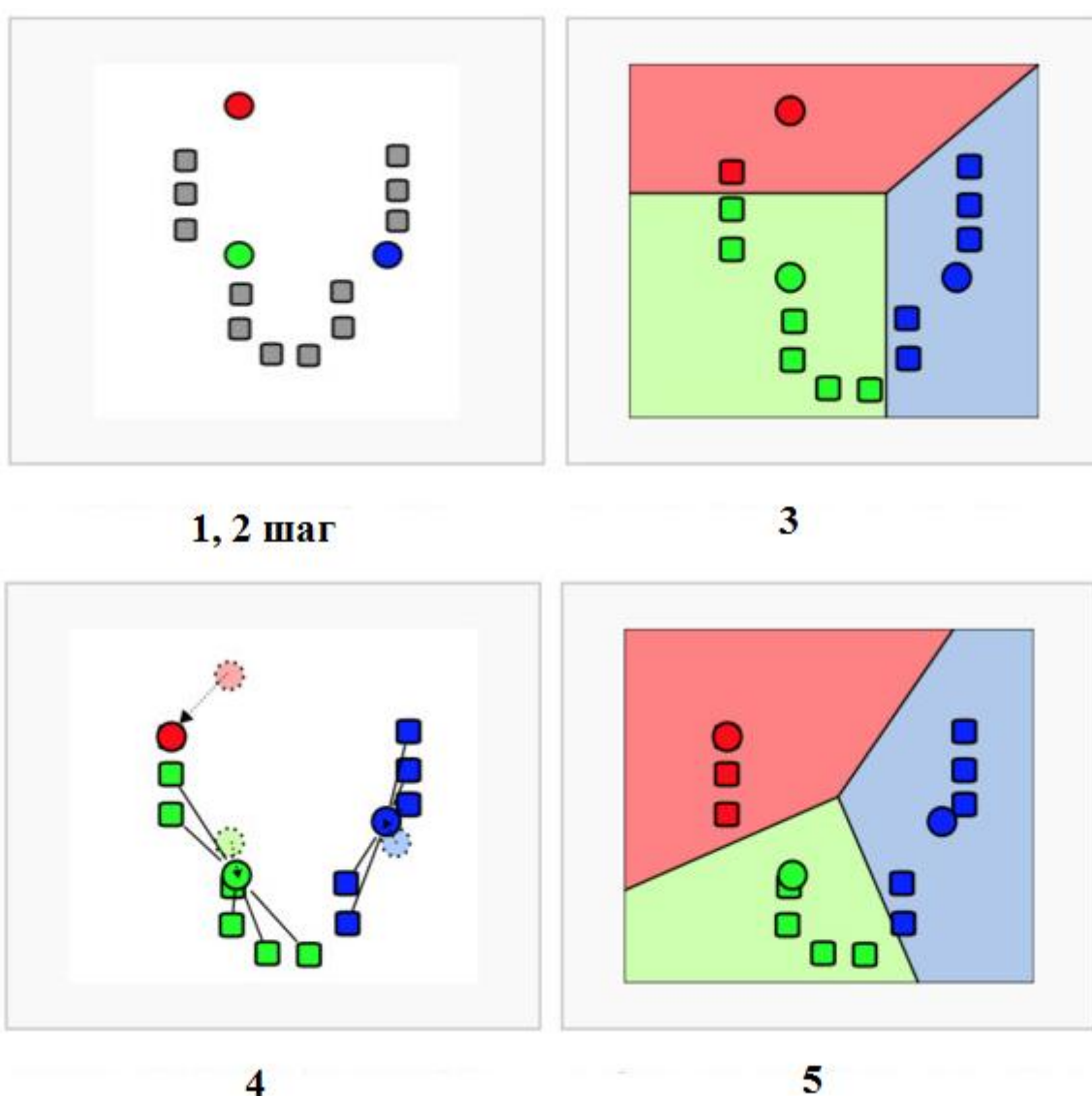
Рис. 9. Визуализация K-средних
