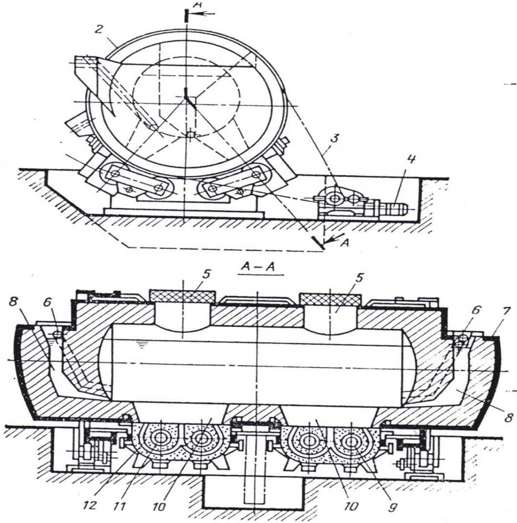
Şekil 1.5. İnduksiya kanal sobası
