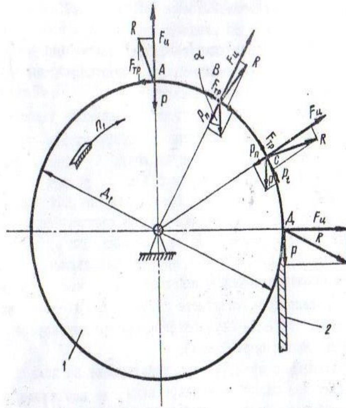
Şəkil 2.2. Fırlanan işçi valikin səthində olan tək – tək uçağanlara müxtəlif qüvvələrin təsir sxemi 1 – işçi valik; 2 – tərpanməz bıçaq
