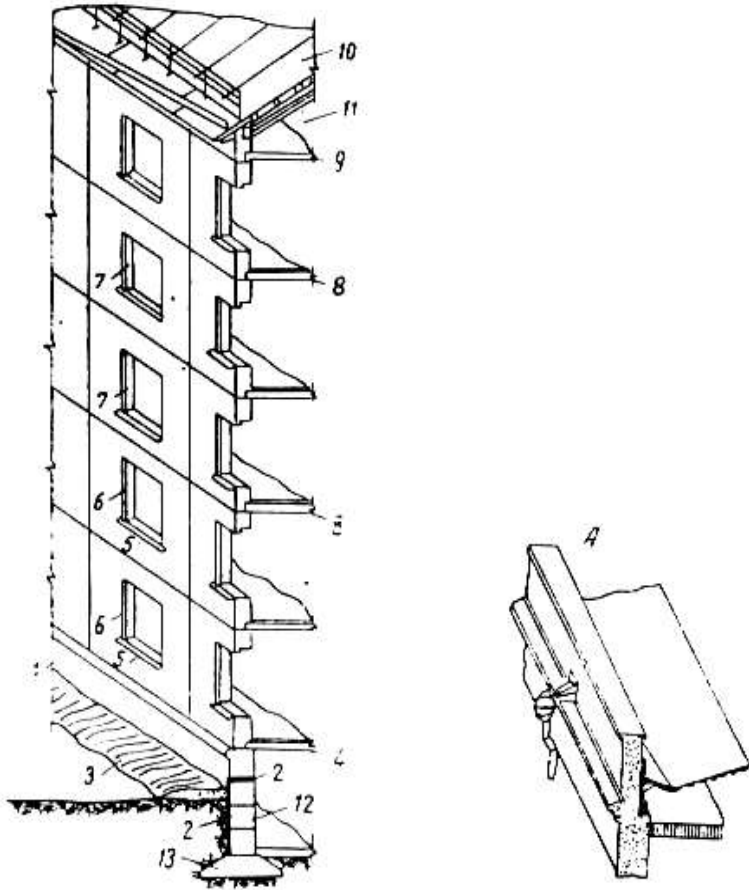
Şəkil 2.4. Yaşayış binasının xarici divarı:
