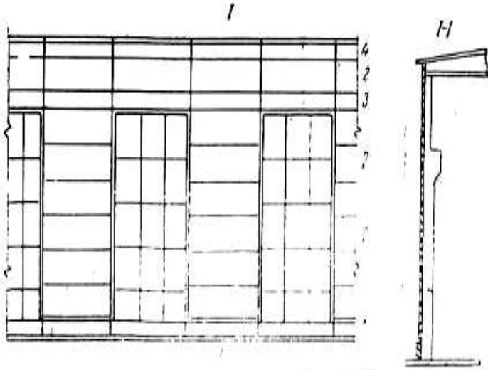
Şəkil 2.15. İri və ağır panellərdən hörülmüş divar. 1-Panelin sokol hissəsi (kürsülük panelləri); 2-Adi cərgə panelləri; 3- Atqı panelləri; 4-karniz panelləri.
