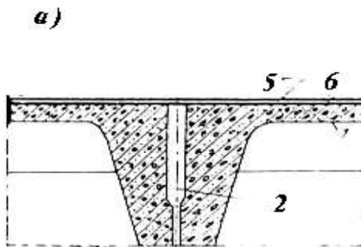
Şəkil 2.16 Örtük konstruksiyası.
