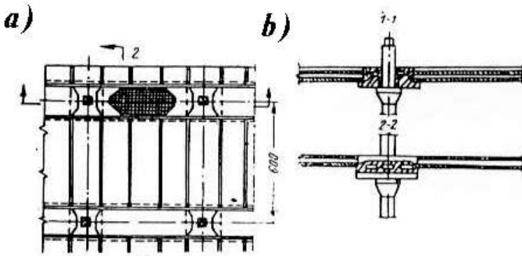
Şəkil 2.8. Yığma monolit tirsiz örtmə: a) plan; b) kəsik.
