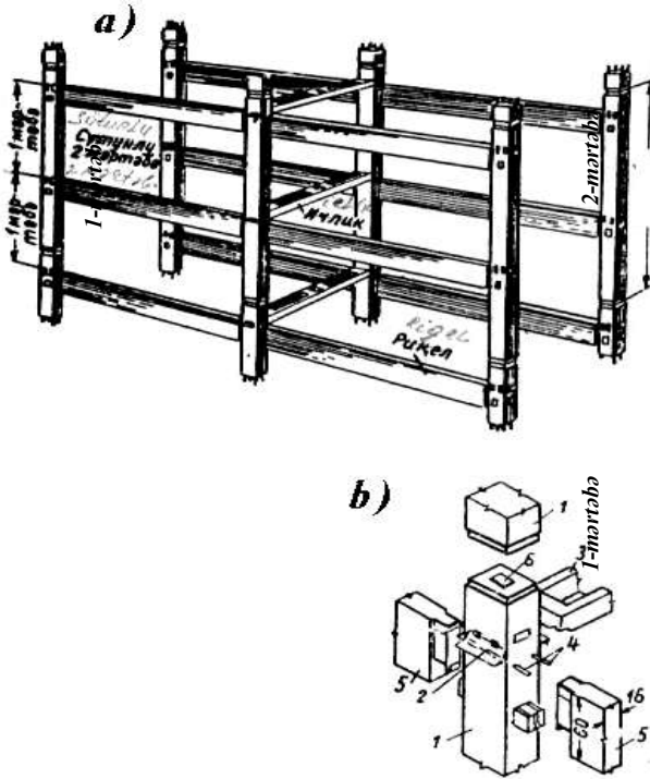
Şəkil 2.5. Yığma dəmir-beton karkas:
