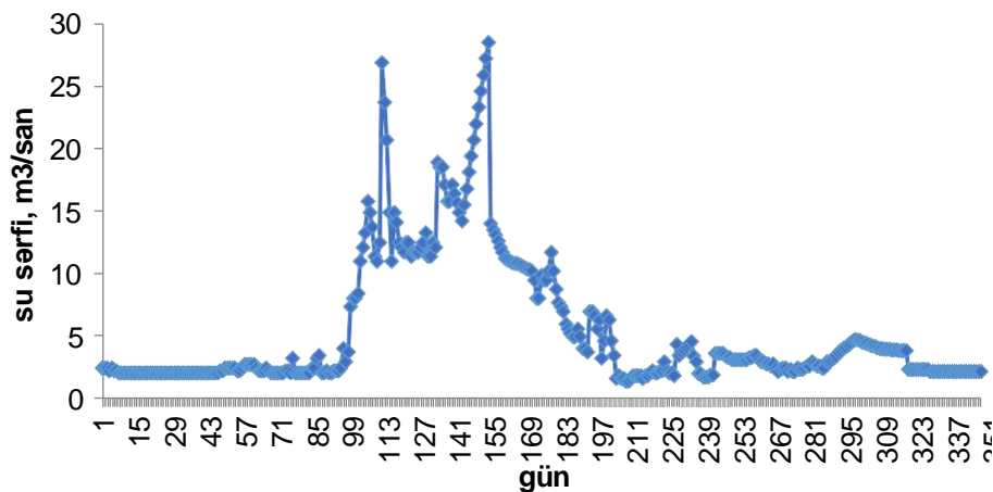
Şəkil 1 - Tərtərçay-Kəlbəcər məntəqəsinin hidroqrafı 1988-ci il üçün
