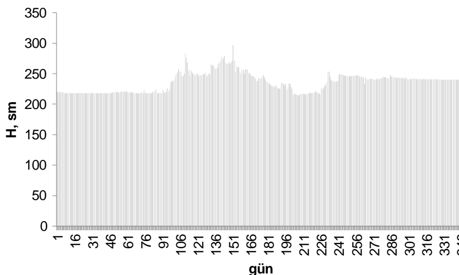
Şəkil 2 - Tərtərçay-Kəlbəcər məntəqəsinin 1988-ci il üçün səviyyə dəyişkənliyi
