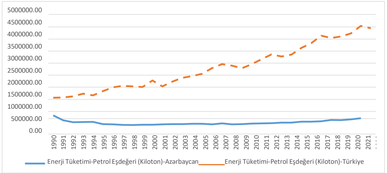
Şekil 5. Azərbaycan ve Türkiye’de Toplam Enerji Tüketimi
