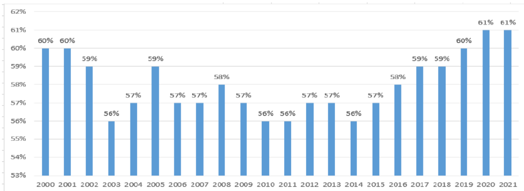
Qrafik 1: Enerji istehlakında müasir bərpa olunan mənbələrin payı, Norveç
