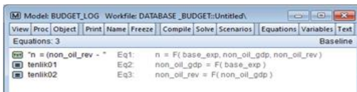
Şəkil 1. İki tərtibli ən kiçik kvadratlar üsulu ilə tənlilər sisteminin həlli (EViews nəticəsi)
