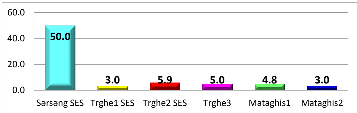
Diaqram 8: Qondarma Dağlıq Qarabağ Respublikasında fəaliyyət göstərən SES-lərin istehsal gücü, MVt-lə
